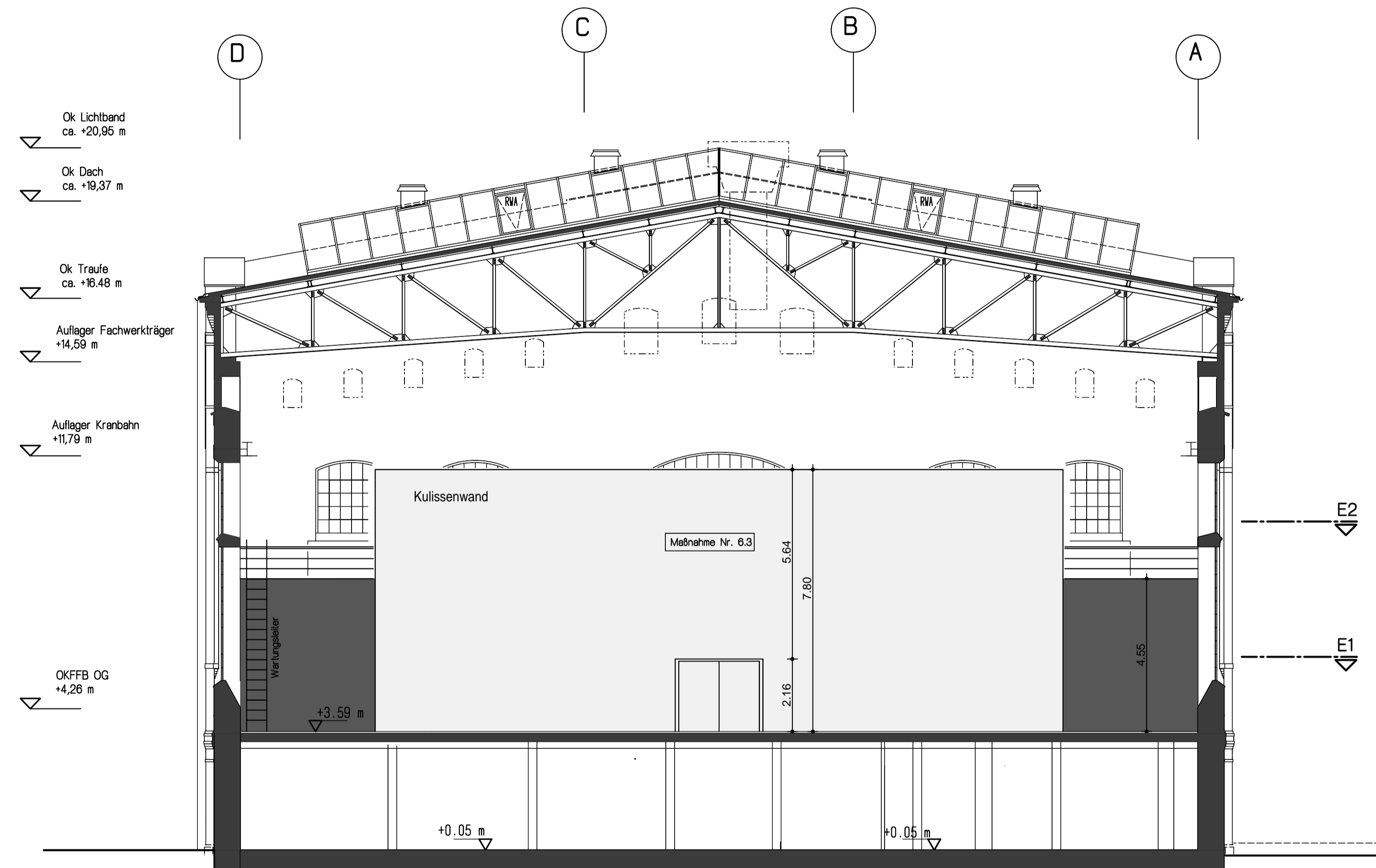
Schnitt SB
