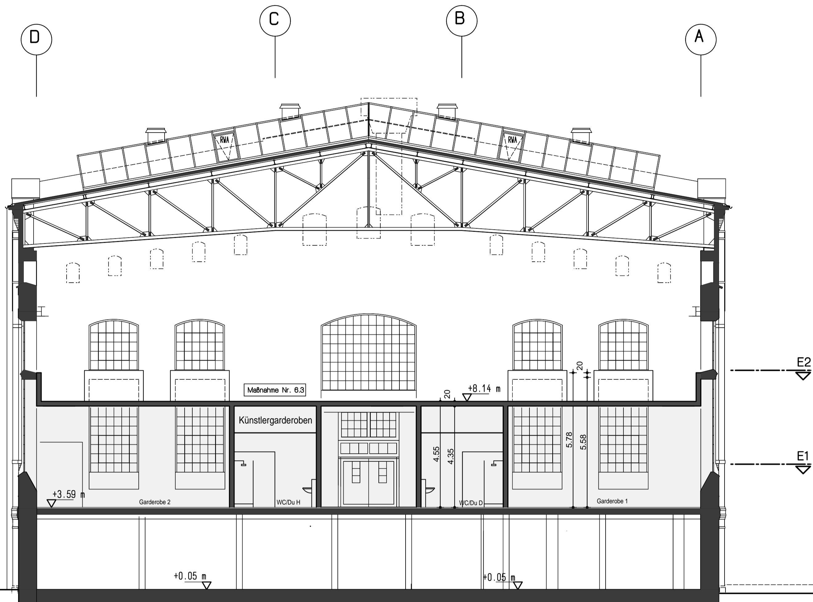
Schnitt SA
